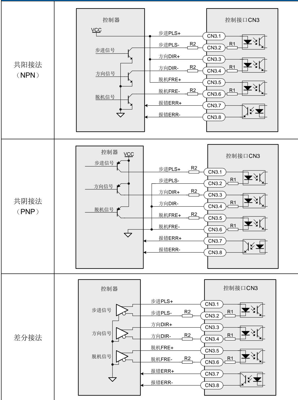
控制接口 CN3 接线示意图
